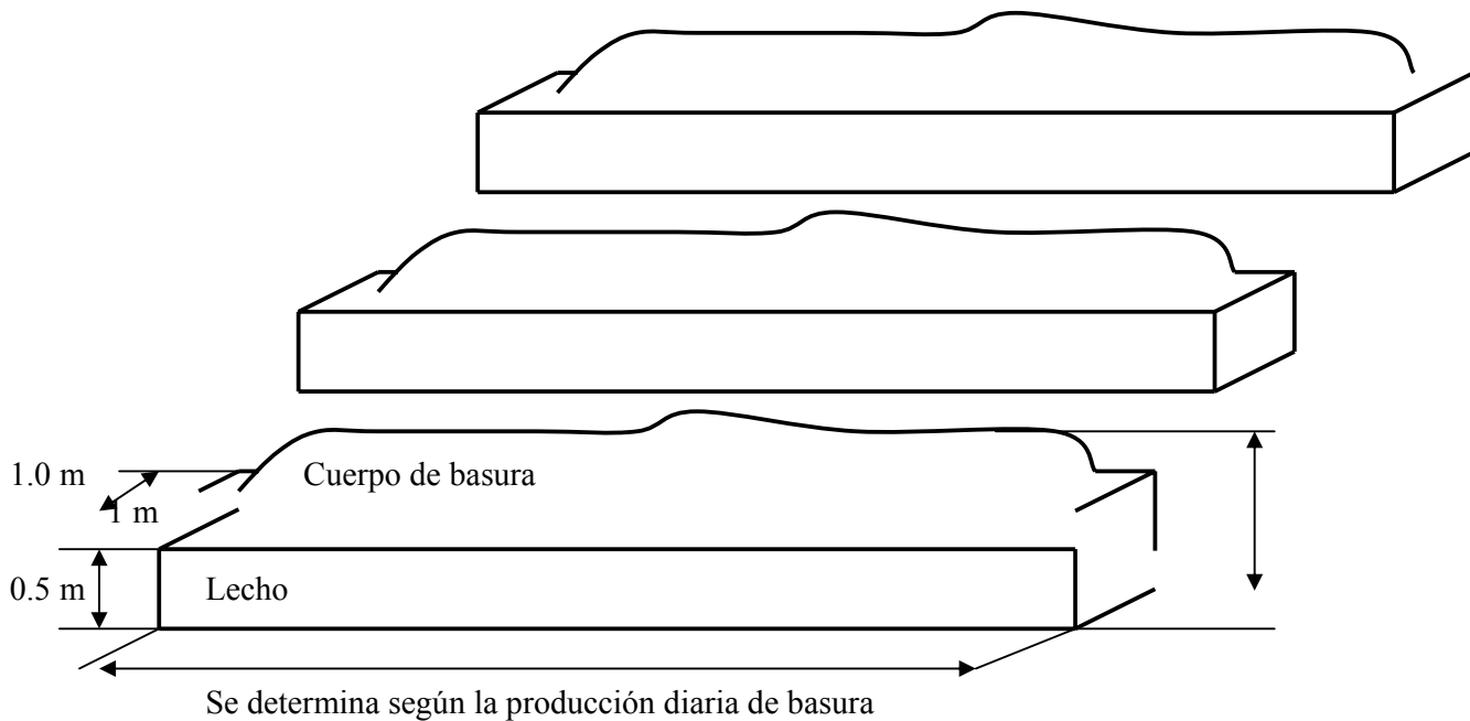
Dibujo 12: Construcción de una planta de lombricultura con lechos.
